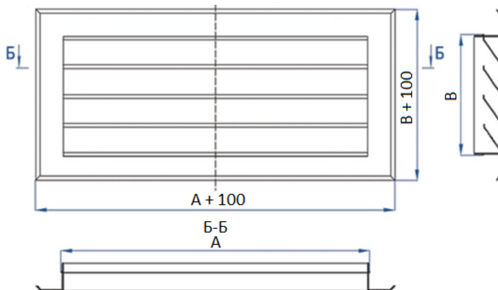
Схема решетки ВР-Н4
